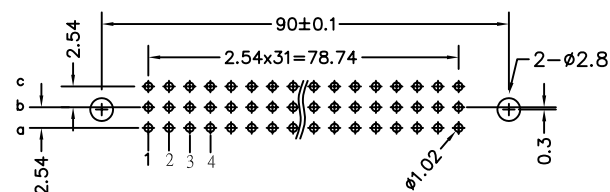
P.C.Board Layout
