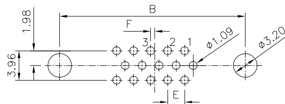
Recommended P.C.B. Layout(15 Pin)
