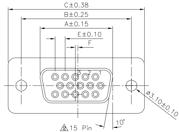
Recommended P.C.B. Layout(15 Pin)
