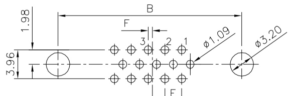
Recommended P.C.B. Layout(15 Pin)
