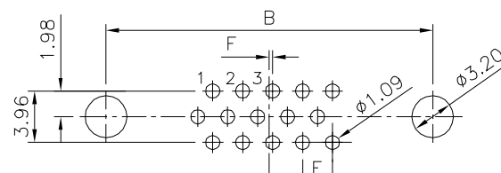
△△ Recommended P.C.B. Layout(15 Pin)
