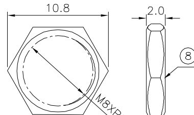
Nut
