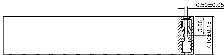
Section A-A
