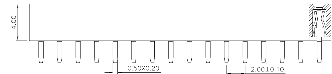
Section A-A
