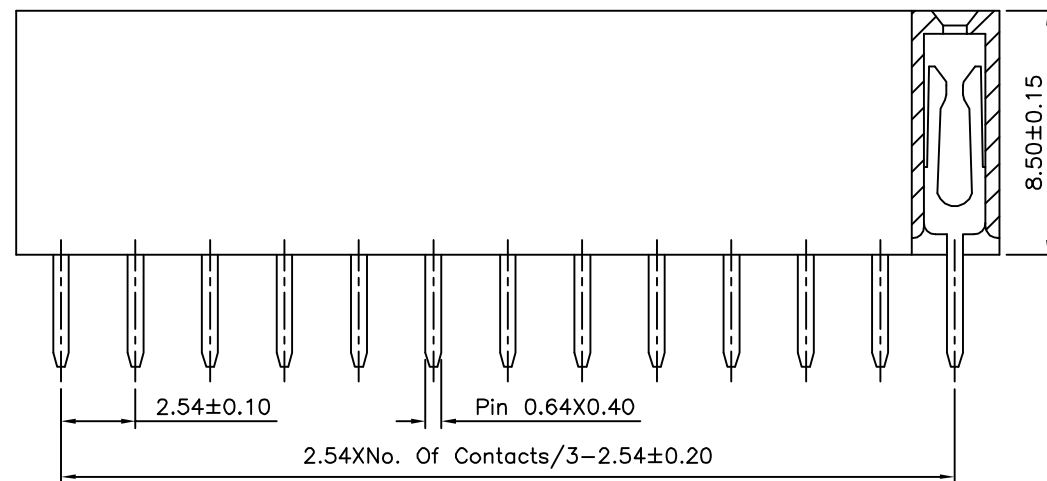
Section A-A
