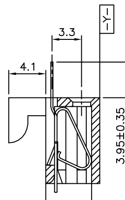
Section:N-N
