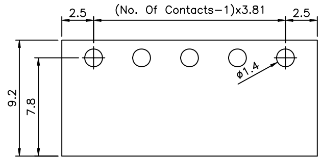
P.C.B Layout
