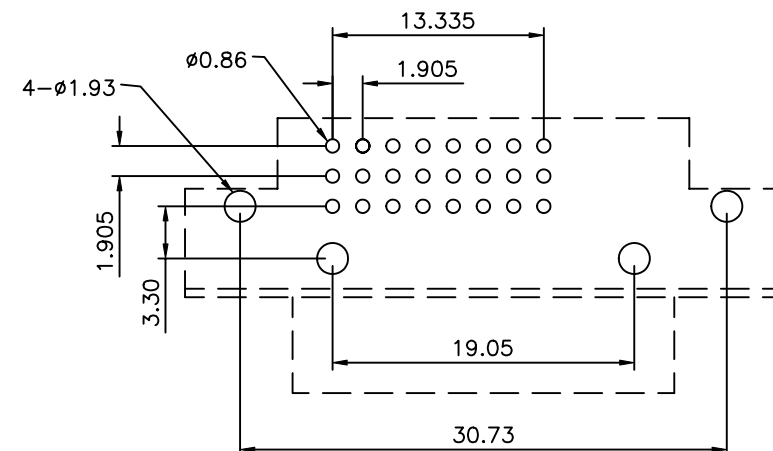
P.C.B Layout
