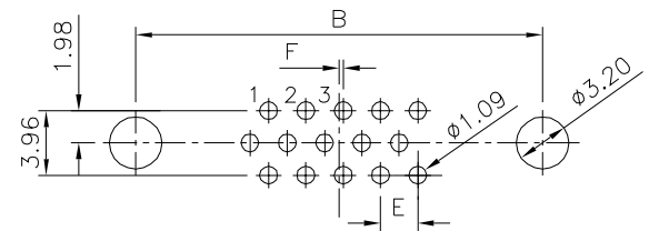
Recommended P.C.B. Layout(15 Pin)
